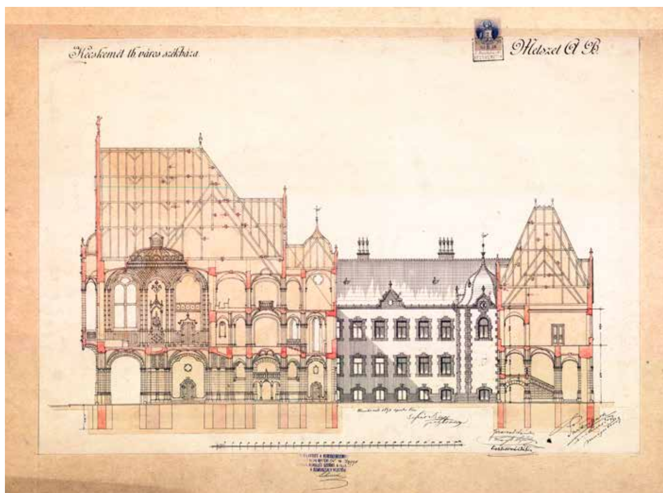
Pártos Gyula – Lechner Ödön: A-B metszet, 1893. április 8. (Magyar Nemzeti Levéltár Bács-Kiskun Megyei Levéltára)
