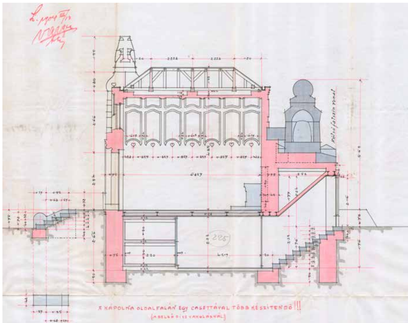
Márkus Géza: A sírkápolna hosszmetsete (1904, Magyar Nemzeti Levéltár Bács-Kiskun Megyei Levéltára)
