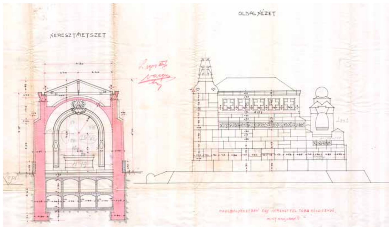
Márkus Géza: A sírkápolna keresztmetszete és oldalnézete (1904, Magyar Nemzeti Levéltár Bács-Kiskun Megyei Levéltára)
