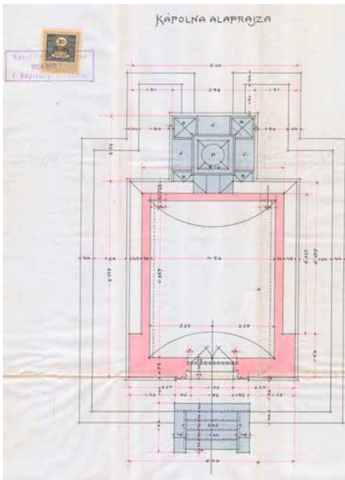
Márkus Géza: A kápolna és a kripta alaprajza (1904, Magyar Nemzeti Levéltár Bács-Kiskun Megyei Levéltára)
