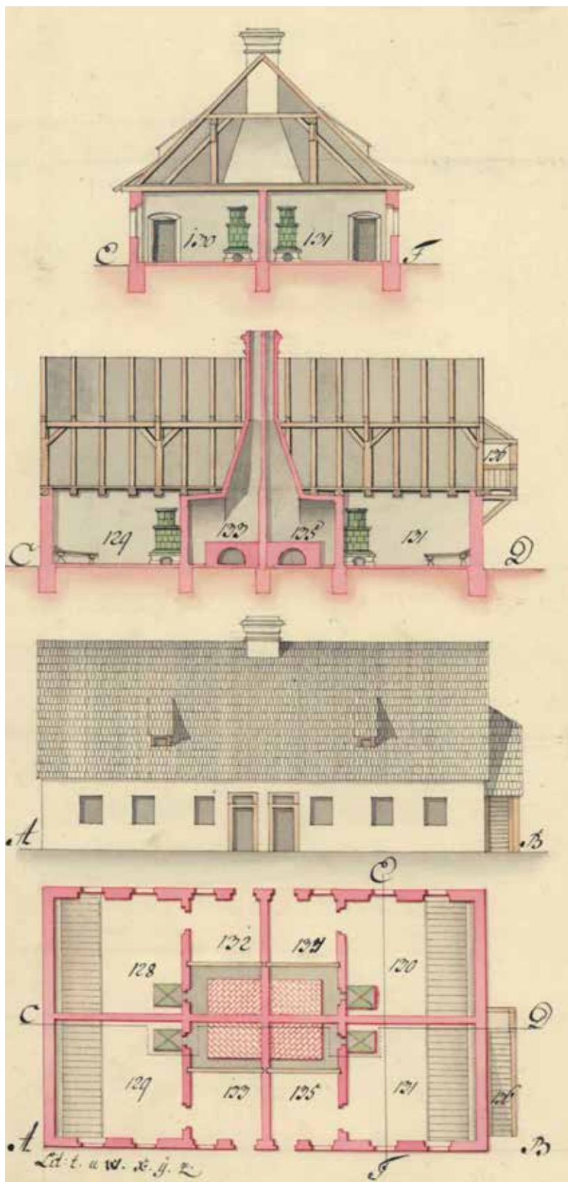
A zimonyi vesztegház egyik négyszobás szállásának oldal- és felülnézeti rajzai (Forrás: MNL OL)
