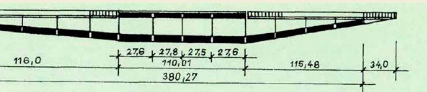
A Szolnoki úti aluljáró hosszszetszeti terve
