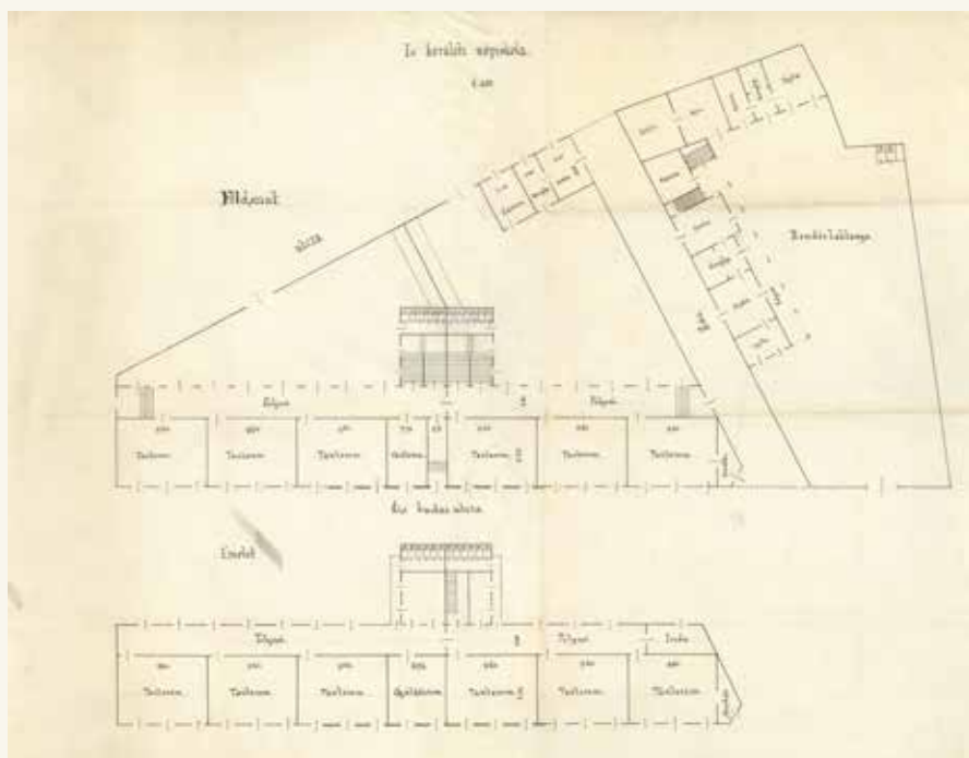
A Budai utcai népiskola alaprajza
