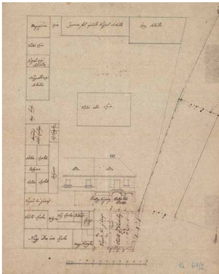
Az Arany Sas vendégfogadó alaprajza, 1830-as évek (MNL Bács-Kiskun Megyei Levéltára)
