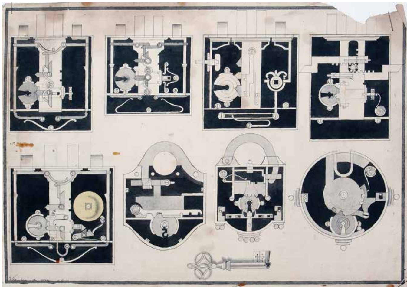
Szűts János zárszerkezet-mintarajzai (1844, Kecskeméti Katona József Múzeum)
