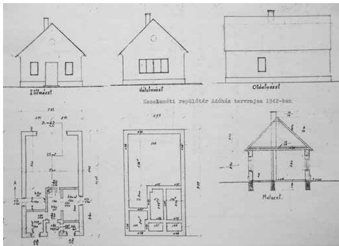
A reptér adóházának tervrajza, 1942
