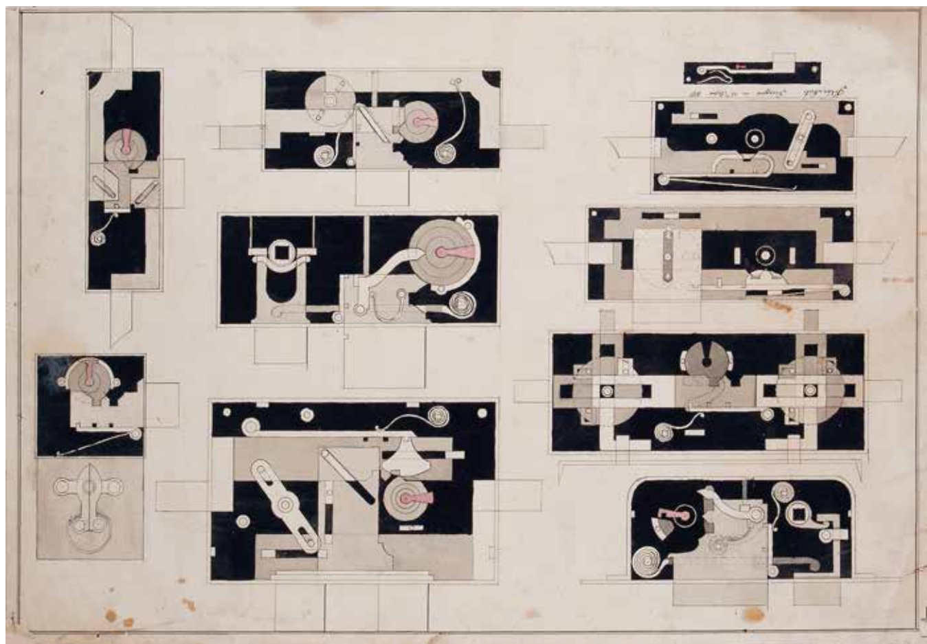
Szűts János zárszerkezet mintarajza (1839, Kecskeméti Katona József Múzeum)
